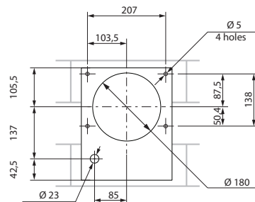
Märkning av hål till enhetens fästeanordningar m.m.
