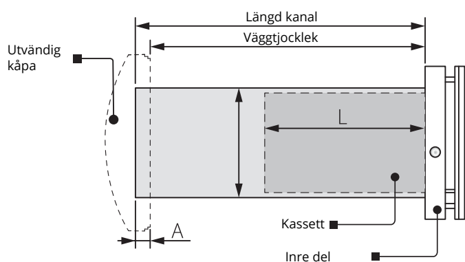
Längd luftkanal [mm]
