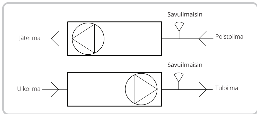
Kaavio laitteen liittämisestä.
