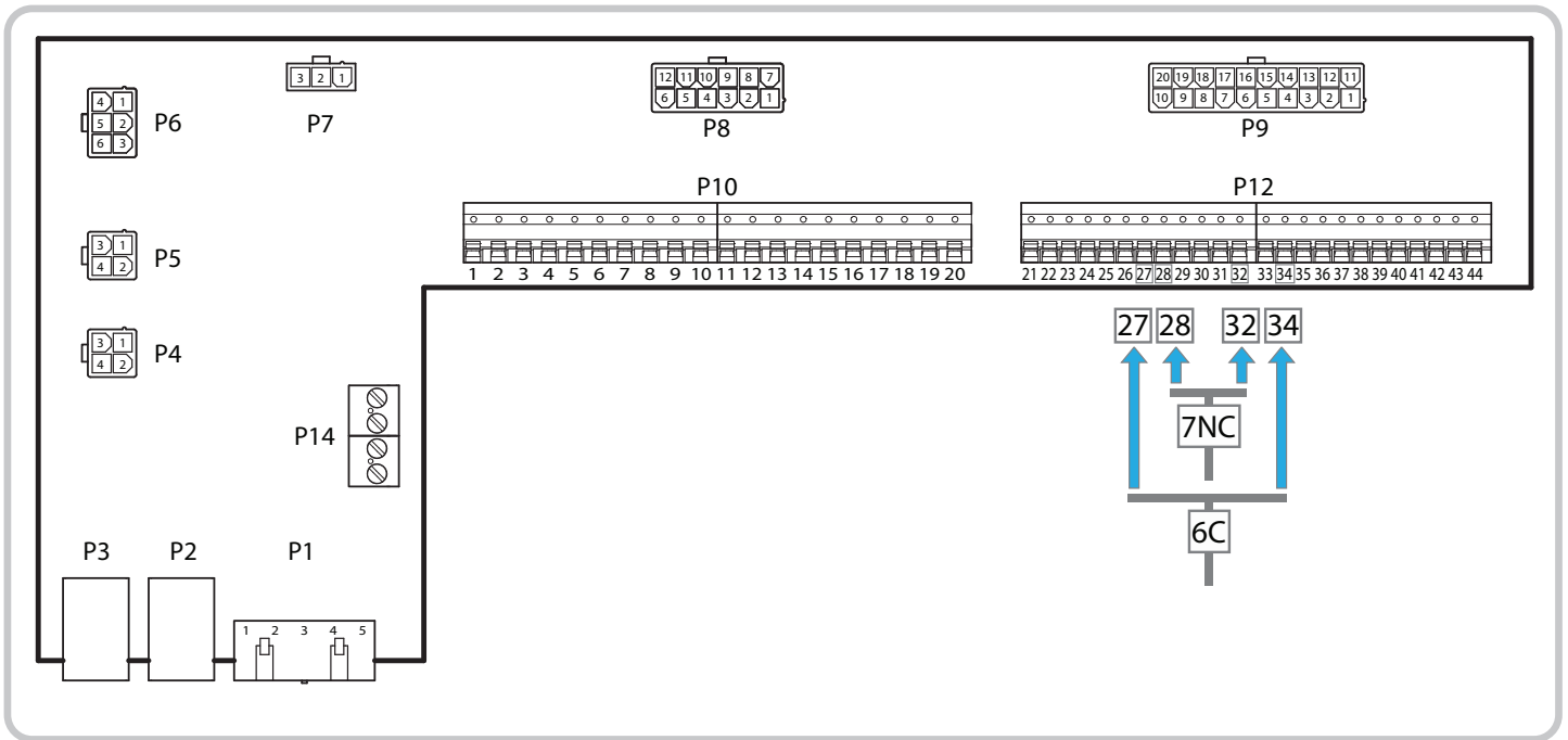
Tilkoblingskort CS2000, CS2500 og CS2500 V2.
