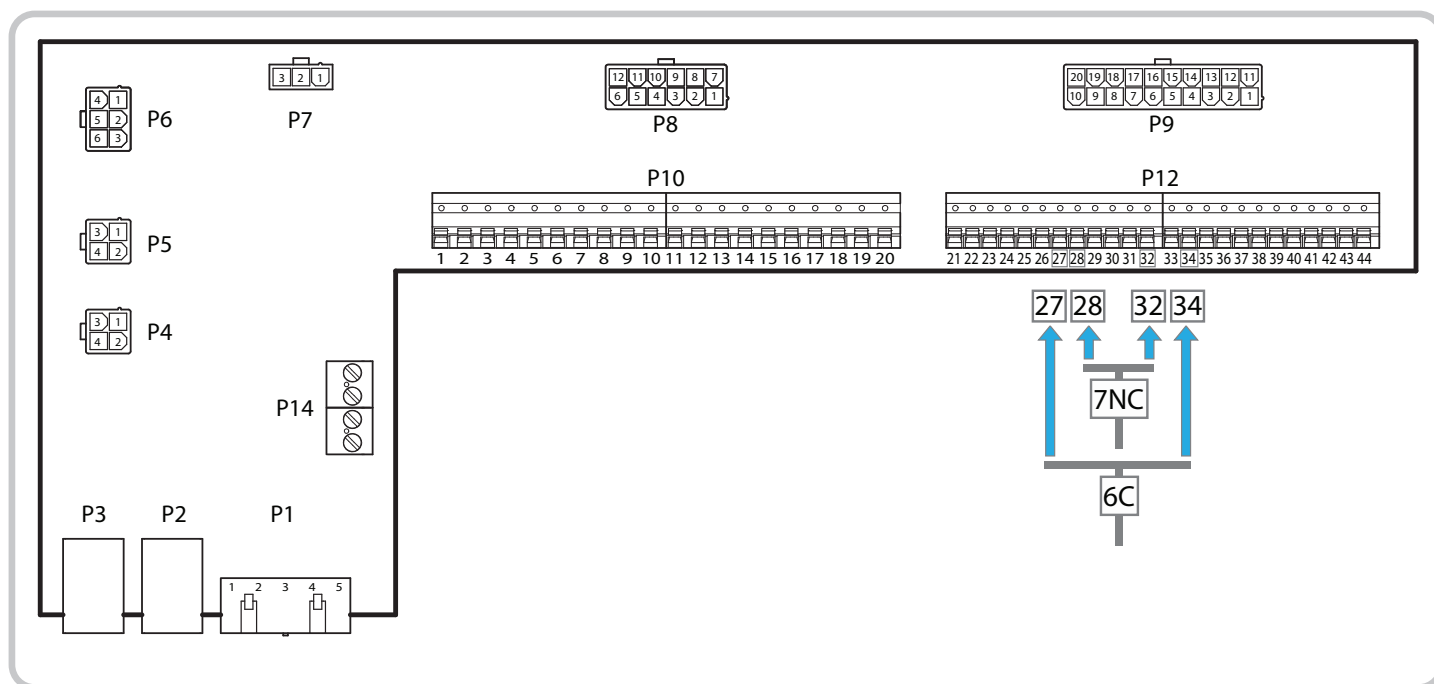
Anslutningskort CS2000, CS2500 och CS2500 V2.
