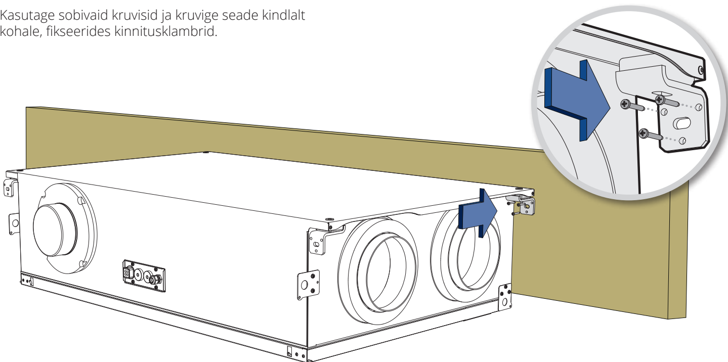
Joonis 10. Külgekinnitus
