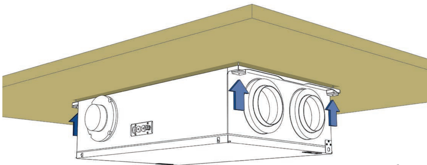
Joonis 8. Ülakinnitus
