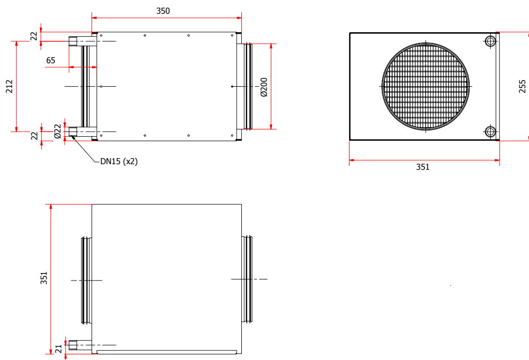
Type D, Ø200, art.nr. 121179
