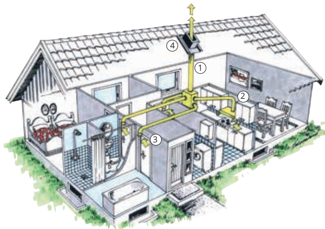
Exempel med frånluftsfläkt ① placerad på vind med frånluft från kök ②, badrum ③ och toalett ④. Frånluften förs till takhuvn över tak.
