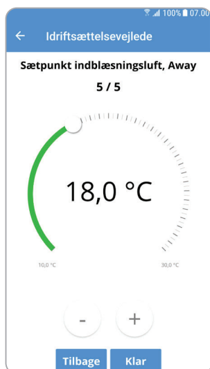
Side 5/5 Indblæsningstemperatur, AWAY
