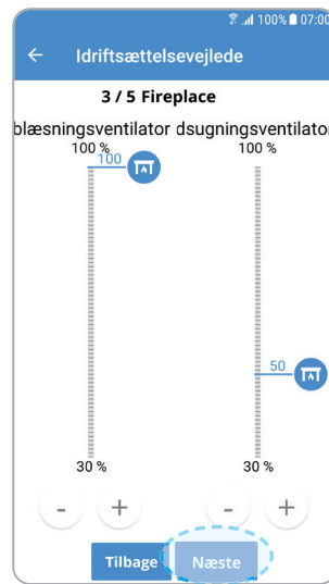
Side 3/5 Luftmængder, FIREPLACE
