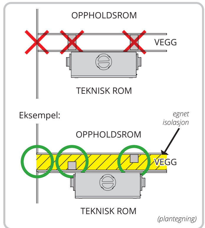
Figur 12 Veggkonstruksjon
