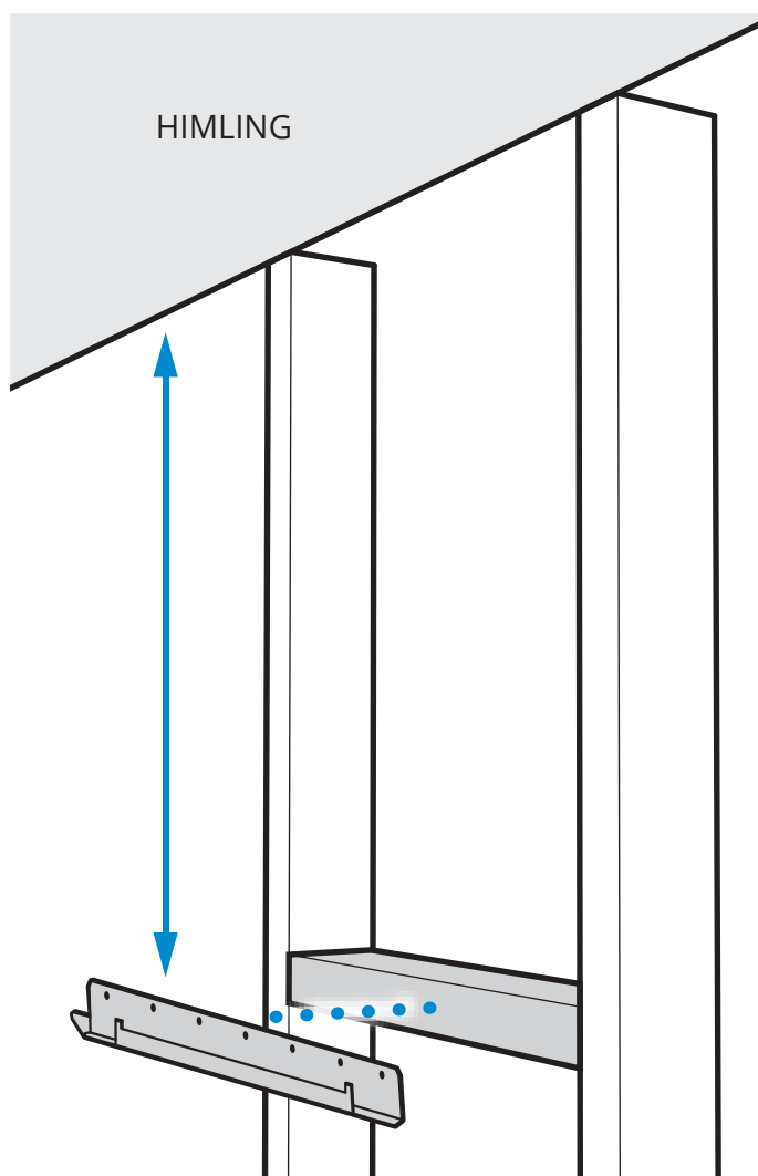
Figur 16 Veggbrakett
